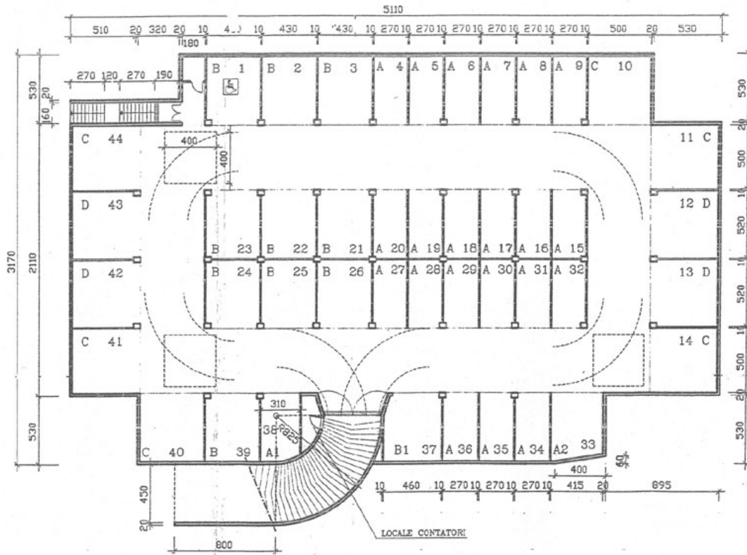
PIANTA PIANO INTERRATO COMPARTIMENTO A
